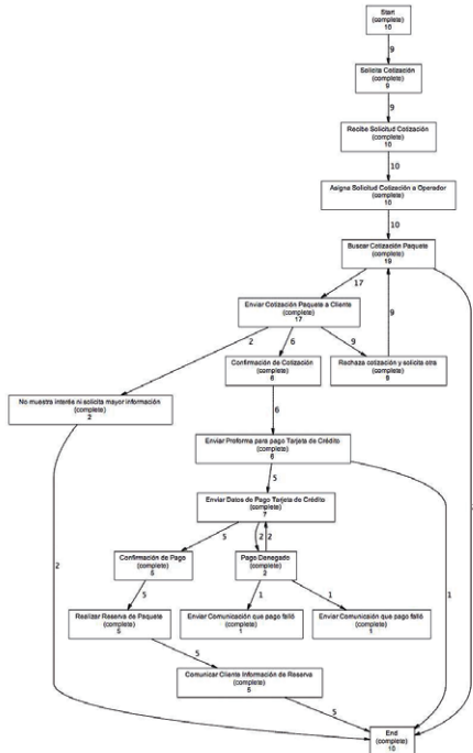
Figura 15. Modelo de proceso descubierto por el Genetic Miner
