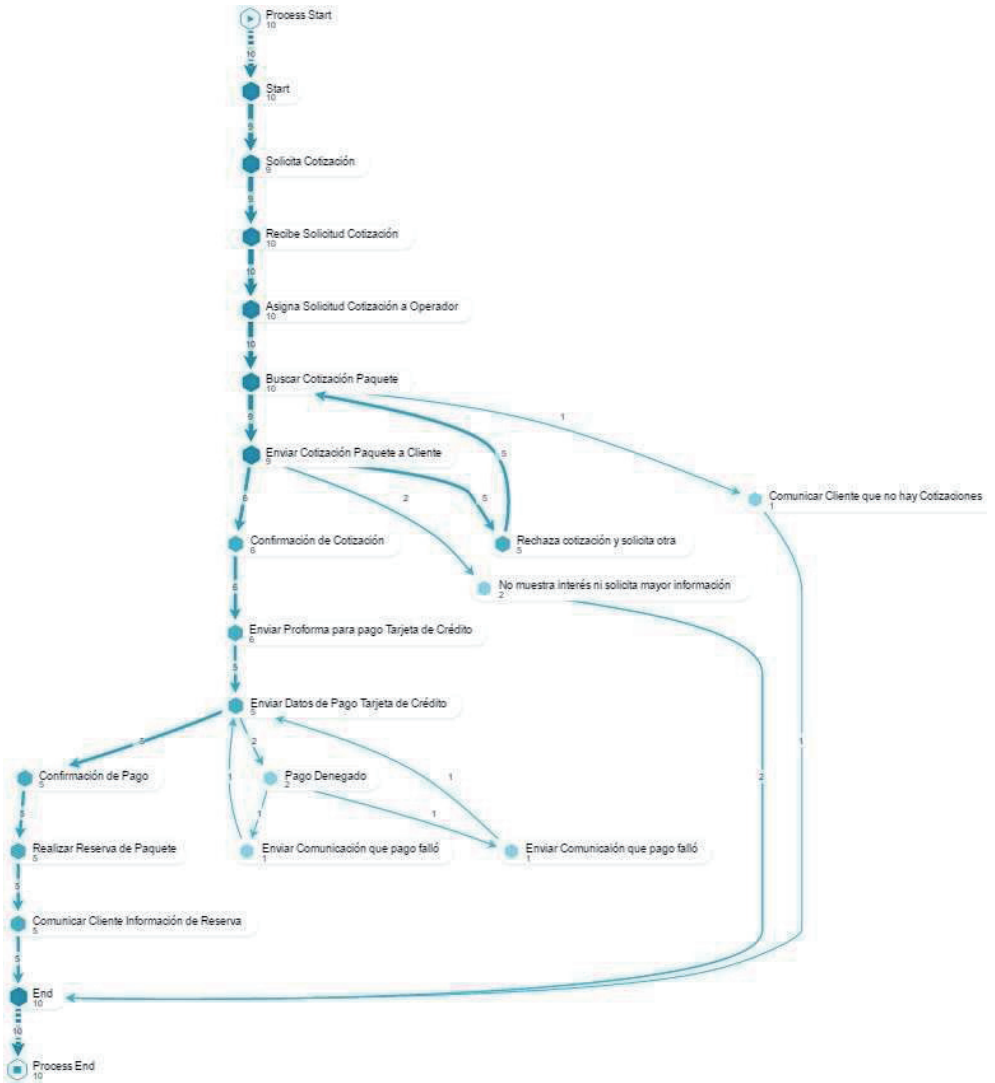
Figura 12. Modelo del proceso con CELONIS Fuente: elaboración propia.
