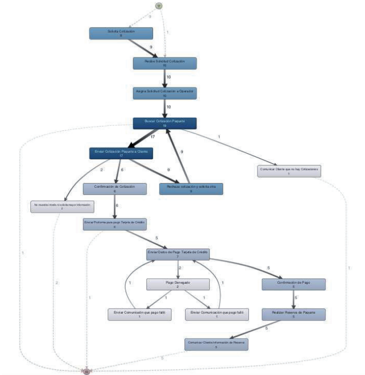
Figura 11. Modelo del proceso con DISCO
