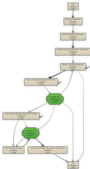
Figura 16. Modelo de proceso descubierto por el Fuzzy Miner
