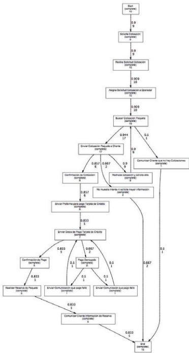
Figura 14. Modelo de proceso descubierto por el Heuristics Miner
