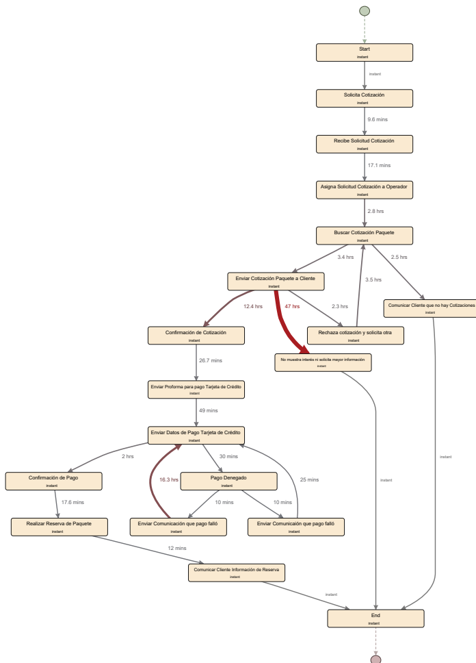
Figura 17. Análisis de desempeño con DISCO
